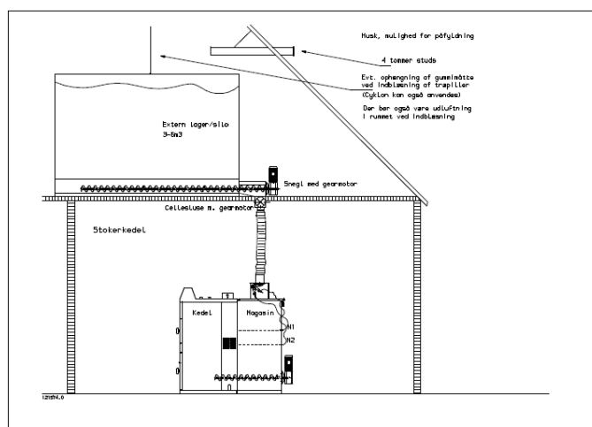
Siloanlæg med etagegennemførelse af transportsystem (ill. BAXI)
